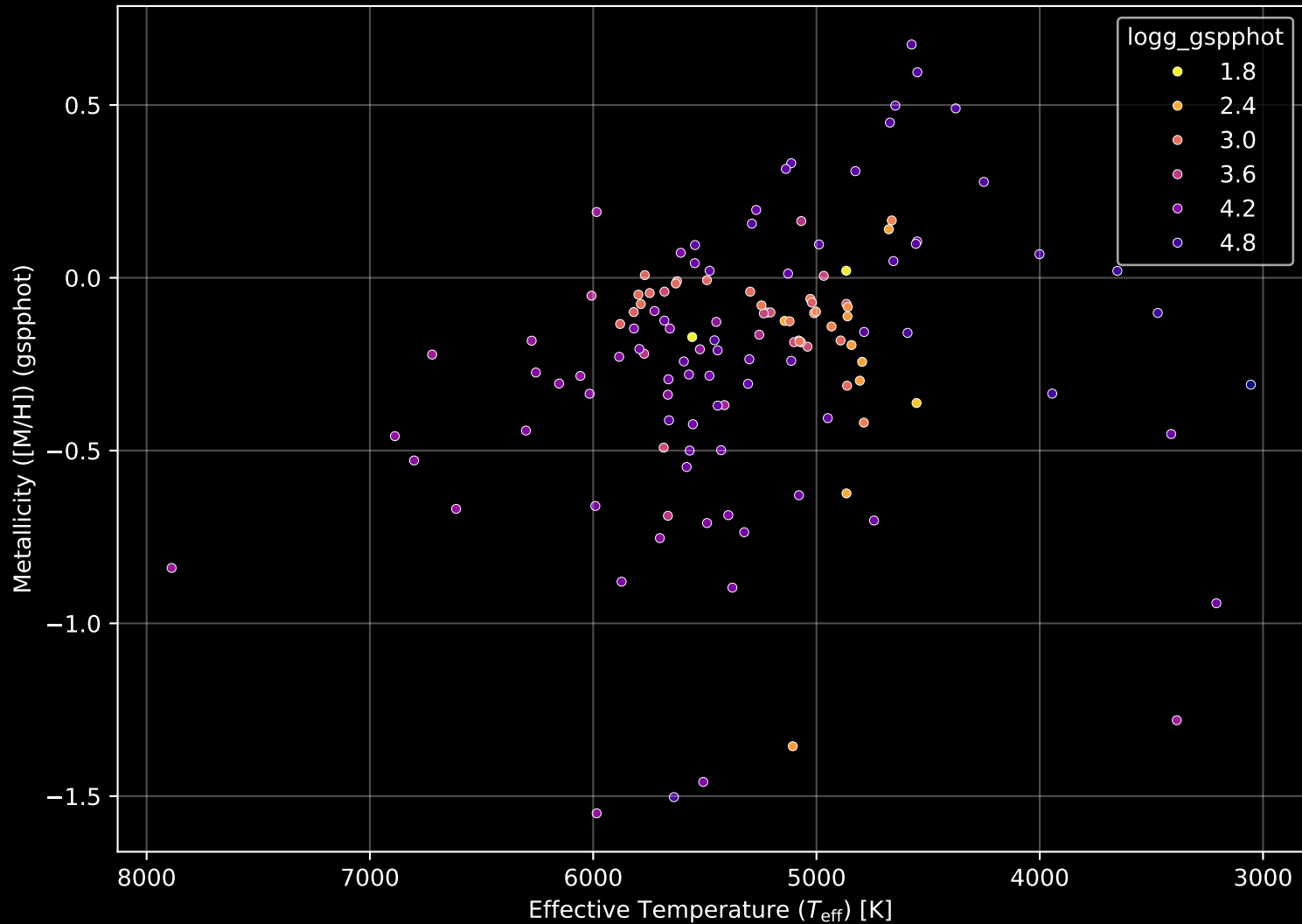
APOGEE DR17 Field: [044+47_MGA] Stellar Population Parameters (n= 130)
